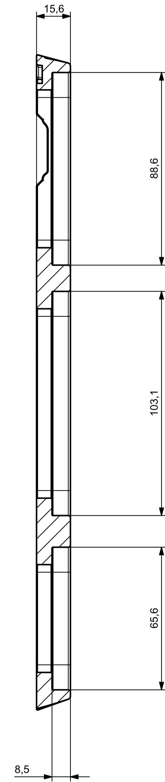
SECTION A-A
